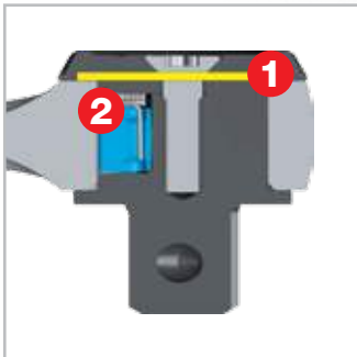
1. Diaframma protettivo 2. Nottolino brevettato
